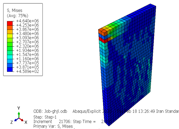
شکل ۹. توزیع تنش فون مایز (S, Mises) در دیوار بنایی بدون تقویت تحت بارگذاری چرخه‌ای.
