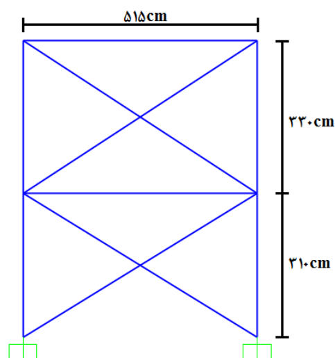
شکل ۱. قاب مورد بررسی
