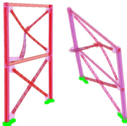
شکل ۹. کمناش خارج از صفحه مهاربند طبقه دوم
