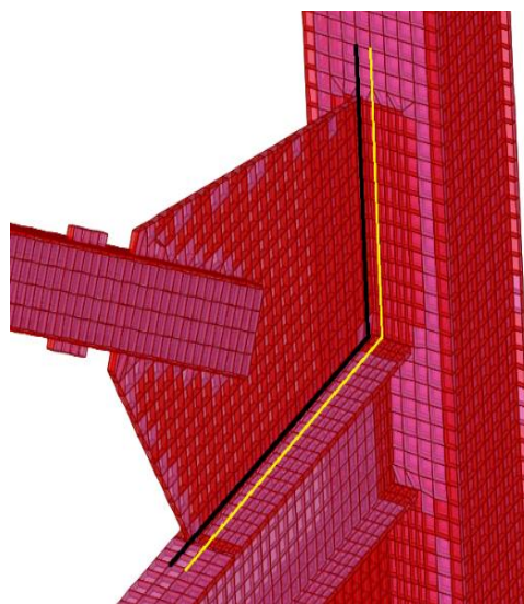
شکل ۵. خروج از مرکزیت خارج از صفحه
